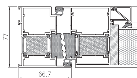
PRZEKRÓJ PRZEZ DRZWI TM 77HI PRESTIGE
