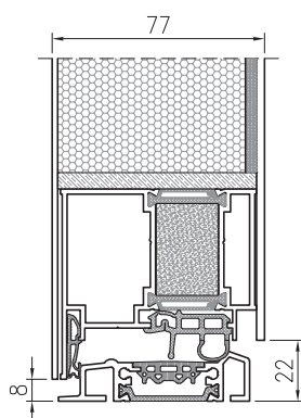
PRZEKRÓJ PRZEZ DRZWI TM 77HI PRESTIGE Z NAŚWIECZEM
