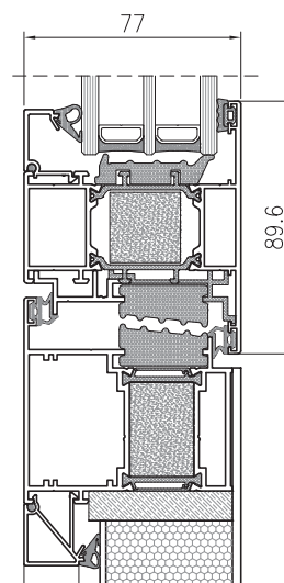
PRZEKRÓJ DRZWI TM 77HI PRESTIGE
