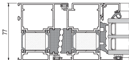
PRZEKRÓJ PRZECZ DRZWI TM 77N HI+ OTWIERANE NA ZEWNĄTRZ
