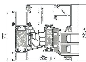
PRZEKRÓJ PRZECZ OKNO TM 77N HI+
