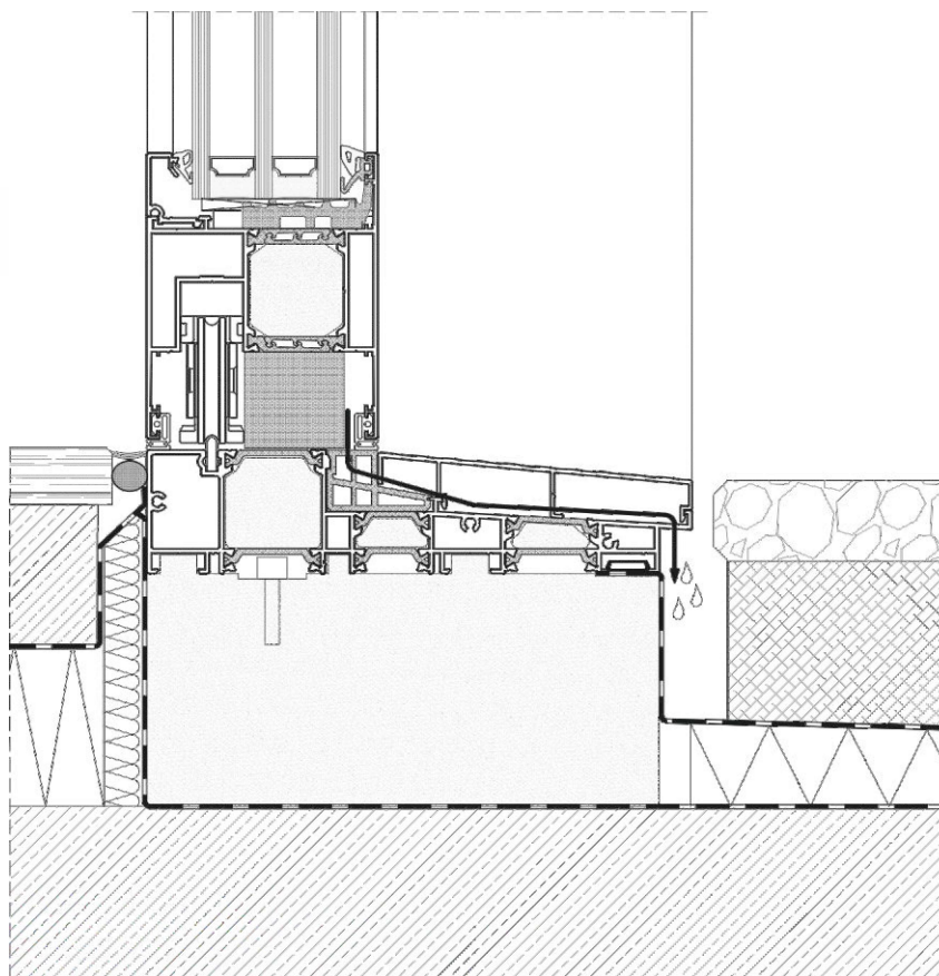
DP 180 PRIMEVIEW PRZĘKRÓJ DOLNY
