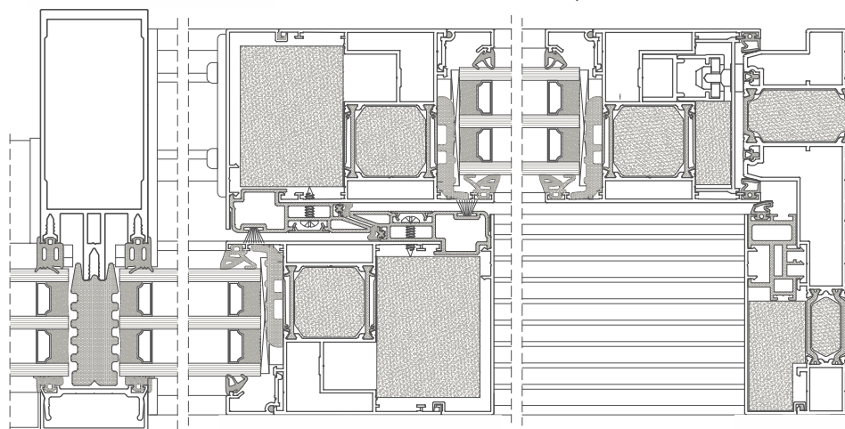
PRZEKRÓJ PRZESZ DRZWI DP180 PRIMEVIEW Z FASADĄ
