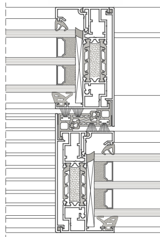
PRZEKRÓJ PRZES SŁUPEK DP 180 PRIMEVIEW
