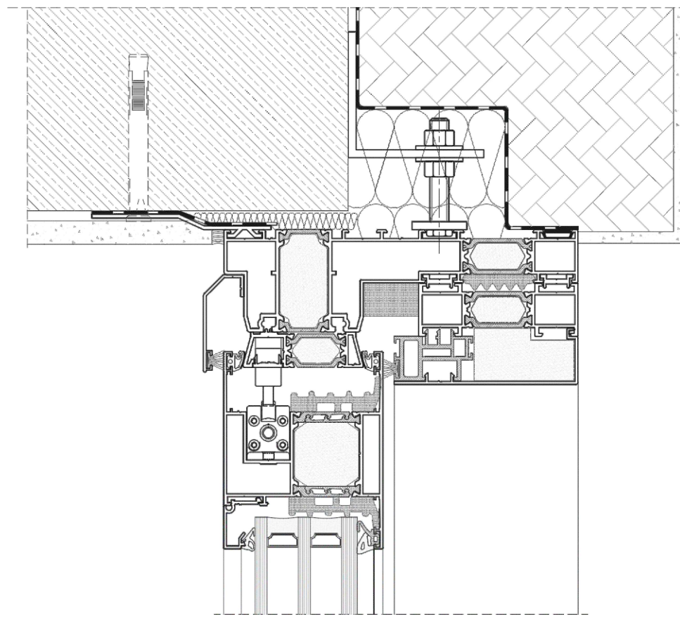
DP 180 PRIMEVIEW PRZĘKRÓJ GÓRNY
