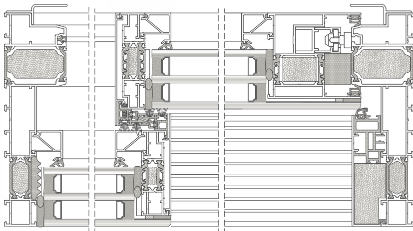
PRZEKRÓJ PRZESZ DRZWI DP180 PRIMEVIEW GLASS
